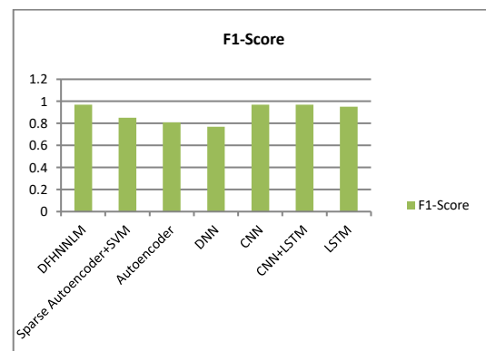
Fig. 5.1.4. F1-Score
