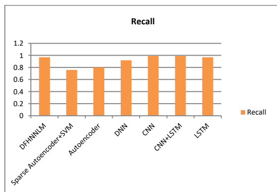
Fig. 5.1.3. Recall
